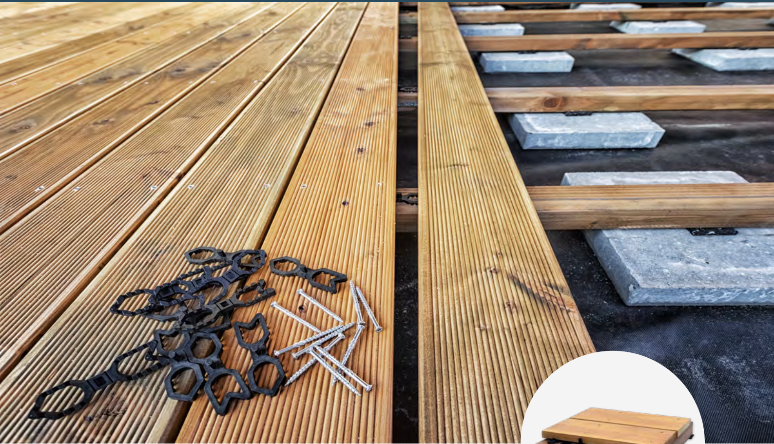
Terrassenzubehörpräsen-ter sichtbare und nicht sichtbare Befestigung gezeigt in einem Modul.
