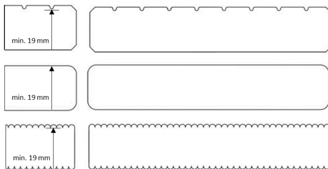
Abmessungen Terrassenprofile - Unterkonstruktion
