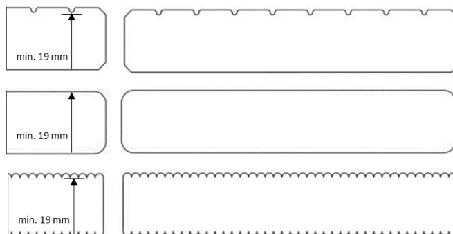
Abmessungen Terrassenprofile - Unterkonstruktion
